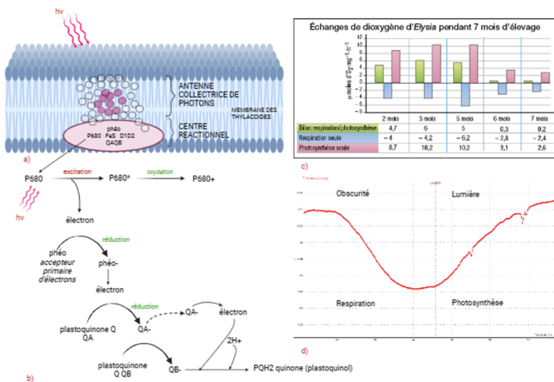
FIGURE 28 – Fonctionnement et rendement quantique de la photosynthèse chez Elysia chlorotica . a) Représentation schématique du photosystème II. b) Le transfert d'électrons à partir de la paire spéciale P680. c) Représentation graphique du rendement quantique de la photosynthèse chez Elysia chlorotica . d) Répartition quotidienne entre la photosynthèse et la respiration.
