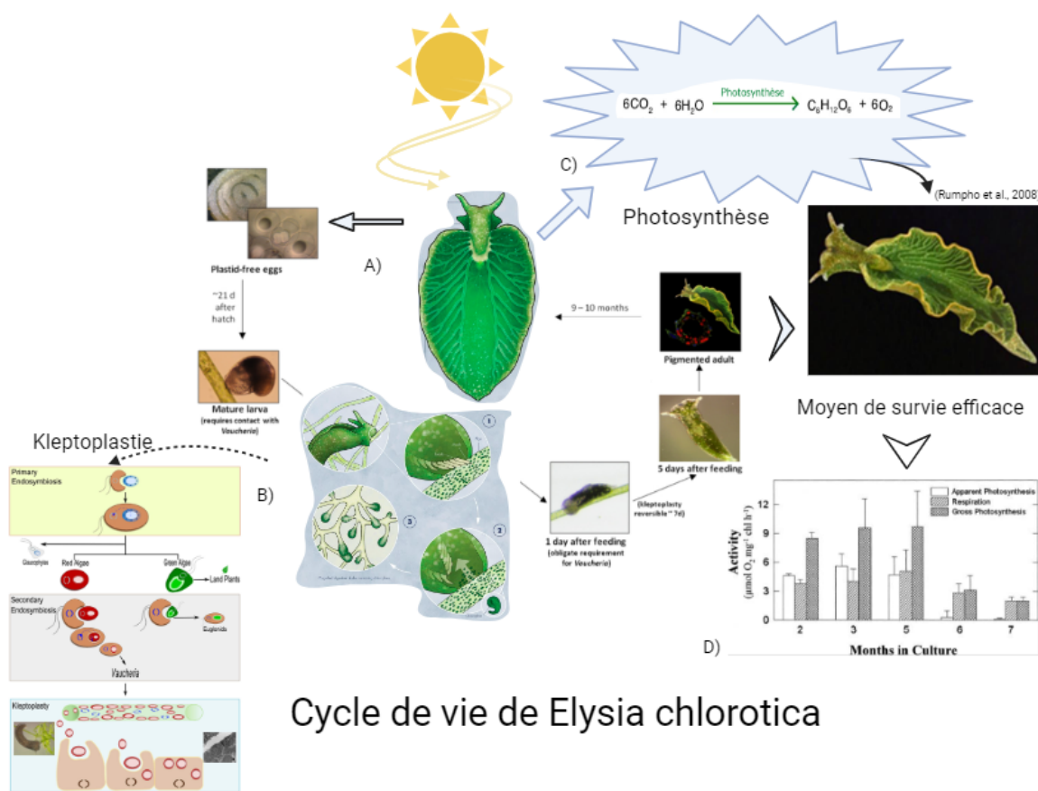
FIGURE 27 – Cycle de vie et acquisition d'un nouveau métabolisme permettant d'effectuer la photosynthèse chez Elysia chlorotica A) Cycle de vie global de Elysia chlorotica . B) Représentation schématique de la kleptoplastie. C) Expression de la capacité à effectuer la photosynthèse chez Elysia chlorotica . D) Représentation graphique de l'activité photosynthétique et respiratoire chez Elysia chlorotica associées en symbiose avec les chloroplastes de Vaucheria litorea et cultivées sur une période de 7 mois en l'absence d'algues.
