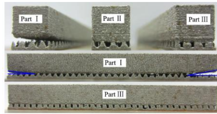
Figure 13. Impact du support sur le gauchissement (Liu, Yang and Wang, 2016)
