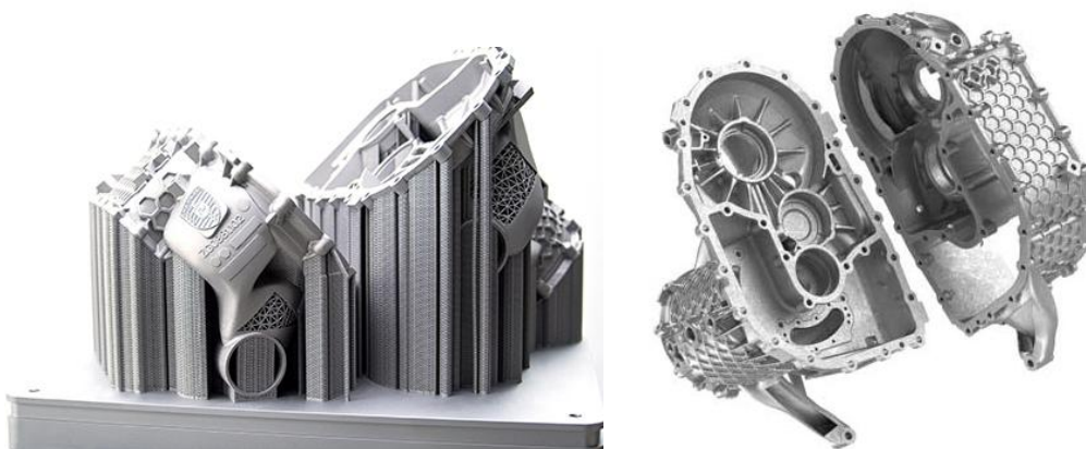
Figure 15. Carter de transmission électrique pour une Porsche, fabriqué par L-PBF, sur le plateau d'impression à gauche et post-traitée à droite. Source : www.slm-pushing-the-limits.com/
