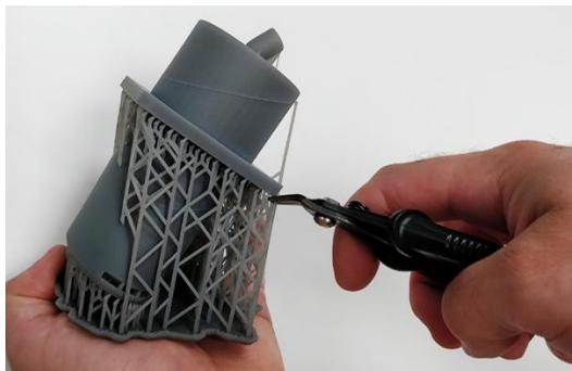
Figure 5 : Exemple d'enlèvement de support et de ponçage sur une pièce imprimée par SLA. Source : makershop.fr
