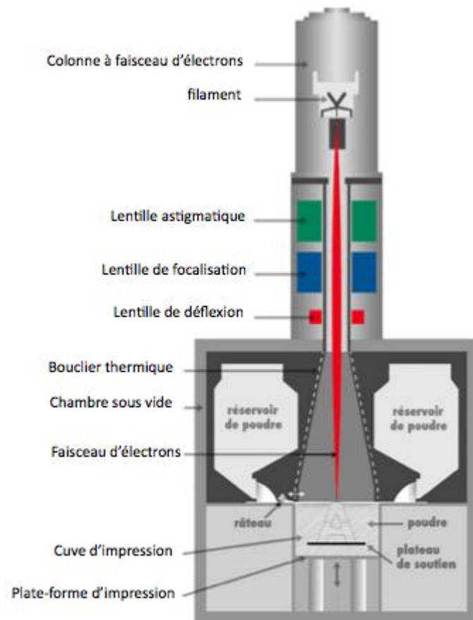
Figure 17 : Schéma de principe de l'EBM
