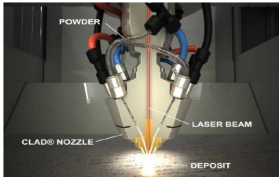
Figure 21 : Vue en écorchée d'une tête de projection CLAD (à gauche) Principe du procédé (à droite). Source : dma-laser.fr
