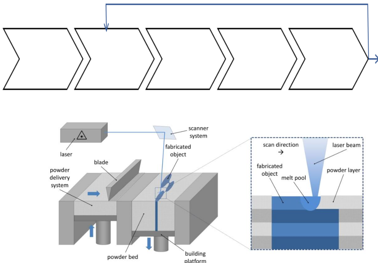
Figure 9 : Principe de la technologie L-PBF (Leitz et al., 2017)
