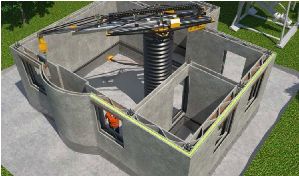
Figure 43 : Construction d'une maison en béton. Source : www.lesimprimantes3d.fr
