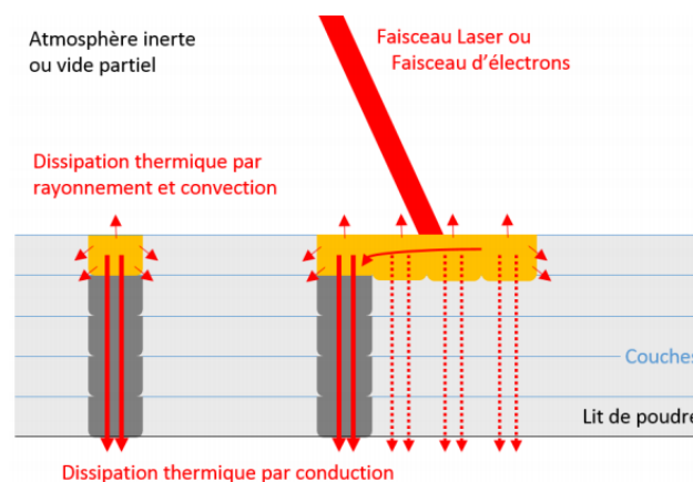
Figure 18 : Exemple de dissipation thermique pour des formes à éviter. Source (Vayre, 2014)
