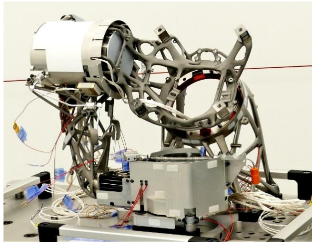
Figure 16. Support de mécanisme de propulsion électrique (ETHM) de satellite, thalesgroup.com
