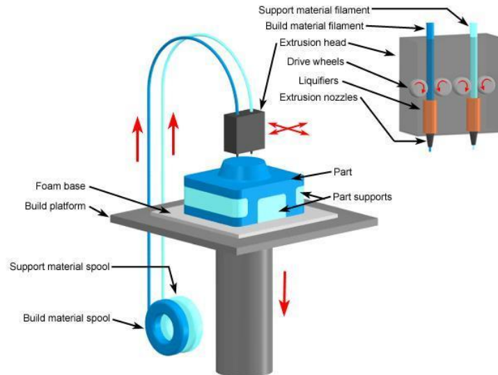
Figure 40 : Principe de l'extrusion de matière. Source : 3Dnatives.com
