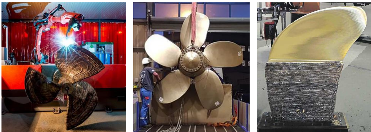
Figure 26 : A gauche, une hélice en cours de fabrication ; Au milieu, hélice installée en 2021 sur un bateau de la marine nationale ; A droite, hélice brute de fabrication en bas et usinée sur la partie haute.
