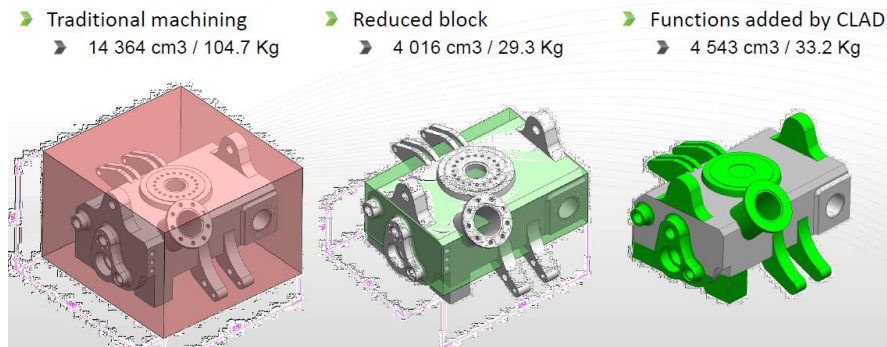
Figure 29 : Rajout de fonctions sur un bloc métallique (Frechard 2015)
