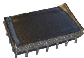
Figure 19 : Déformations géométriques à cause du trop faible nombre de supports (structures cylindriques sous la pièce) (Vayre, 2014)
