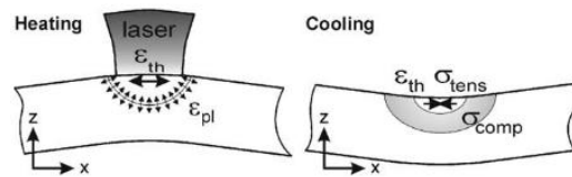
Figure 12. Gauchissement de surface (Kruth et al. , 2004)
