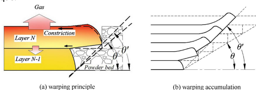
Figure 11. Déformation plastique des surfaces en porte à faux dû au gauchissement (Wang et al. , 2013)
