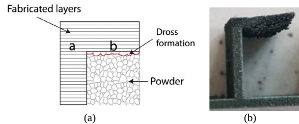
Figure 10. (a) Scories sur surface en porte à faux pour LBM (Calignano, 2014); (b) Mise en évidence du phénomène de scorie lors d'impression de porte à faux (Imprimé sous LBM par MAQ-3D)
