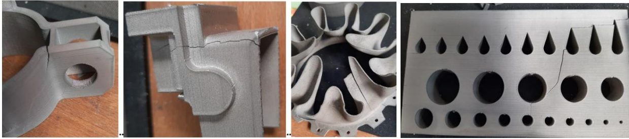
Figure 31 : Divers exemples de pièces fissurées suite au frittage
