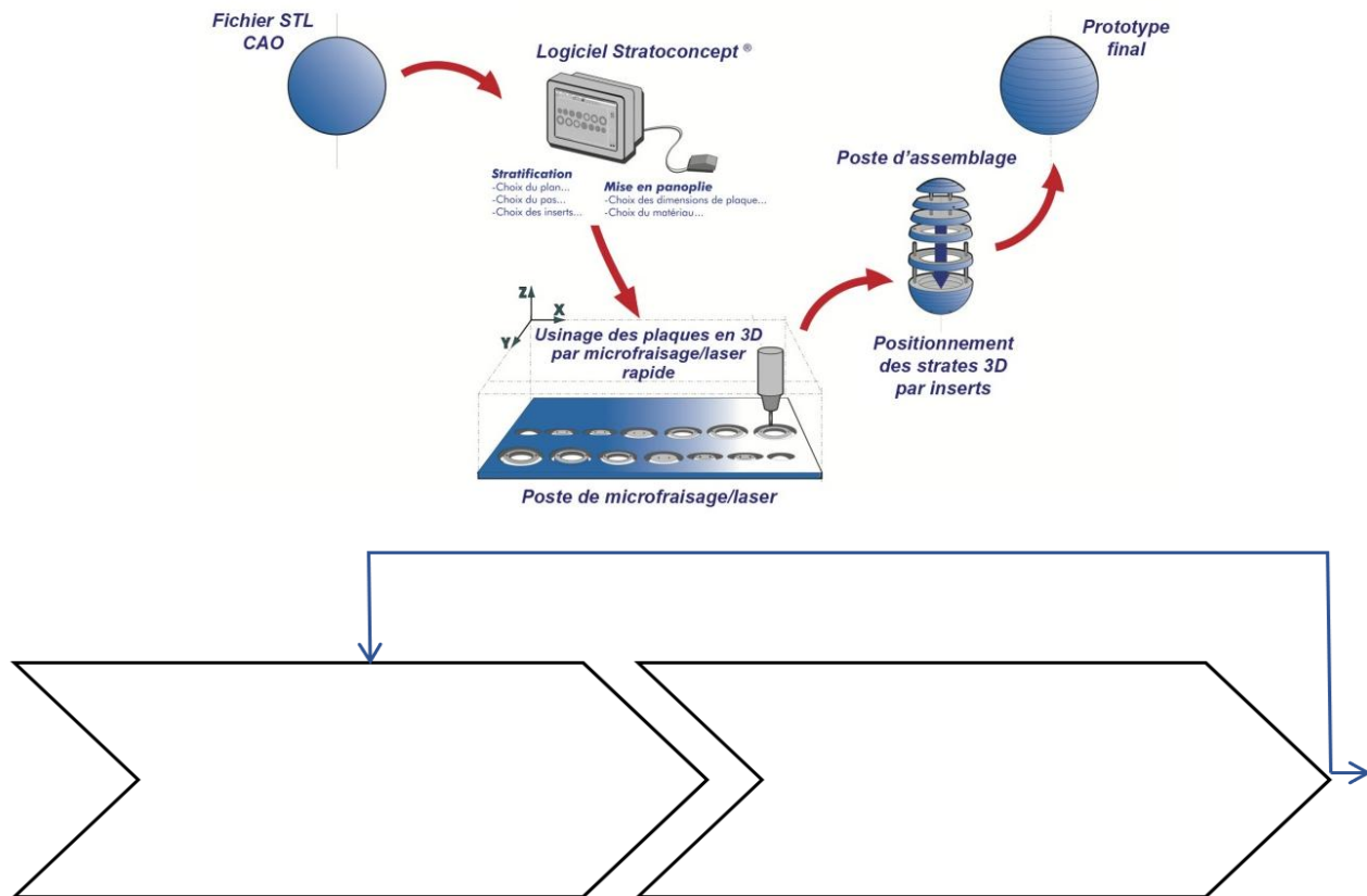
Figure 37 : Principe du procédé. Source http://www.stratoconception.com
