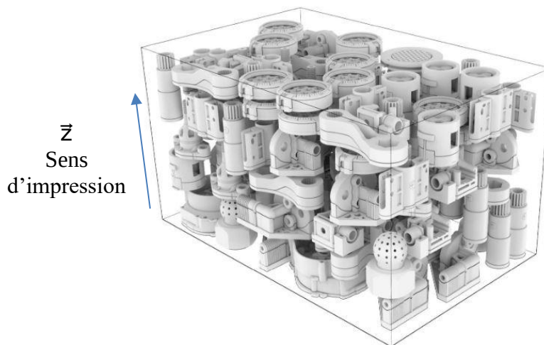
Figure 35 : Des centaines de pièces peuvent être imprimées par lots en même temps. Le logiciel de l'imprimante aide à imbriquer les pièces dans le volume total de la capacité de l'imprimante. (Source : Desktop Metal)
