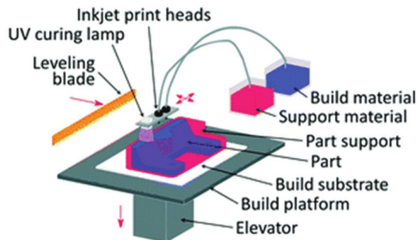
Figure 46 : Principe de la MJM. Source http://prismadd.com
