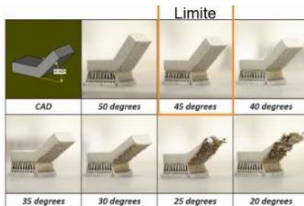
Figure 14. Angles limites (à gauche) ; Supports nécessaires pour la fabrication
