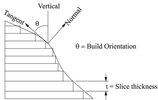
Figure 3 : Staircase effect (l'effet escalier) du procédé de dépôt de couche (Pandey, Reddy and Dhande, 2007)
