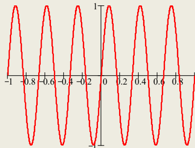
Fonction : y = \sin(6\pi t)
